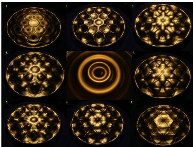
Fig. 1 Ciclu de metamorfoze geometrice ale suprafeței de undă realizate în lichide volatile (etanol) la o frecvență de 14 Hz, având aspectul unui vechi simbol mediteranean numit generic Floarea vieții
